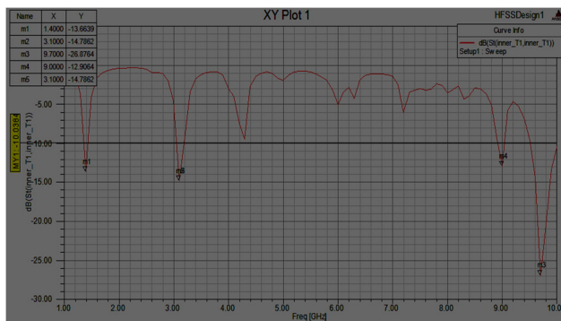
Fig 5: S11 Parameter Vs Frequency
