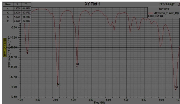
Fig 4: S11 Parameter Vs Frequency
